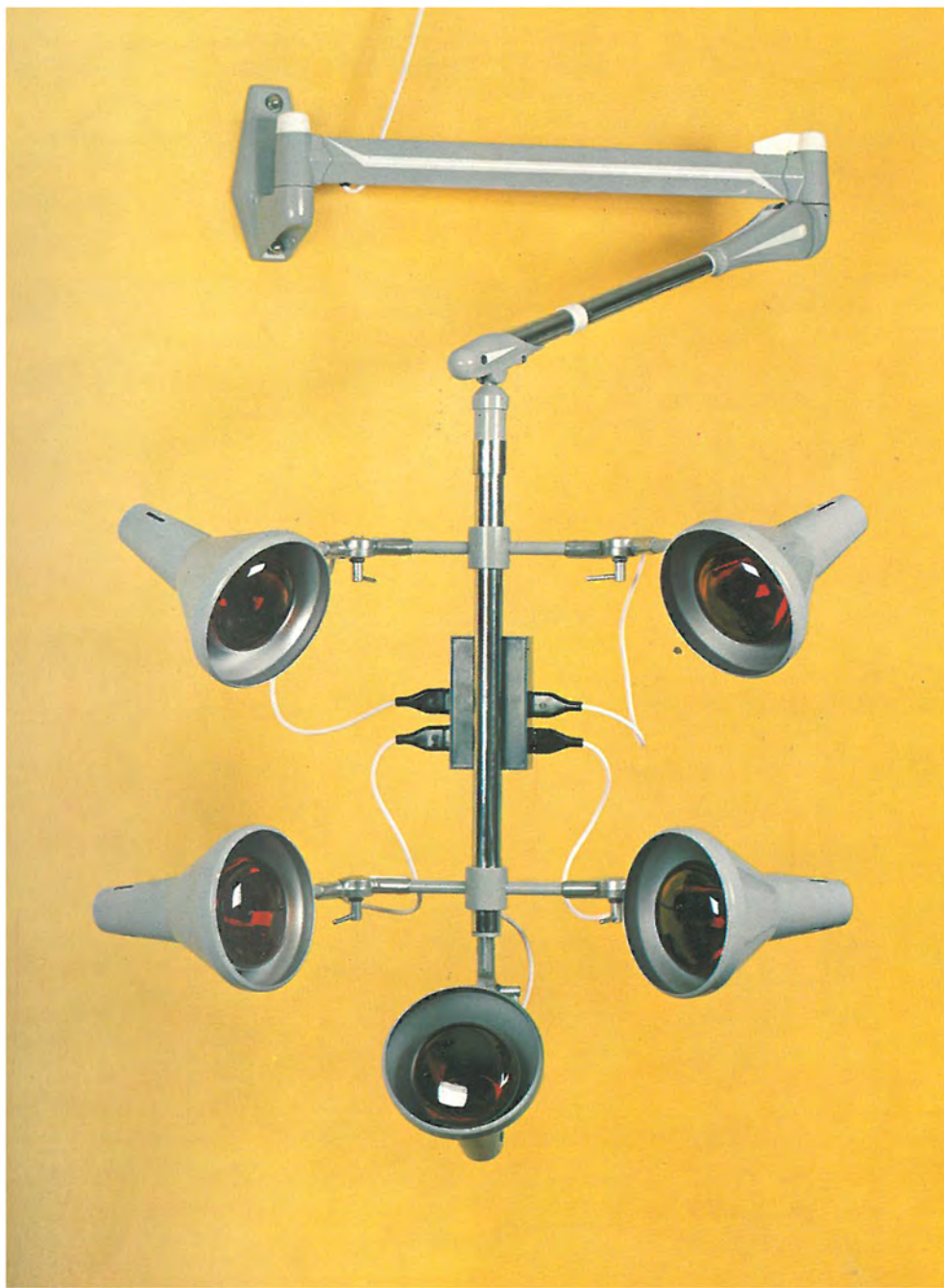
Complesso murale con 5 lampade a raggi infrarossi Euromatic
